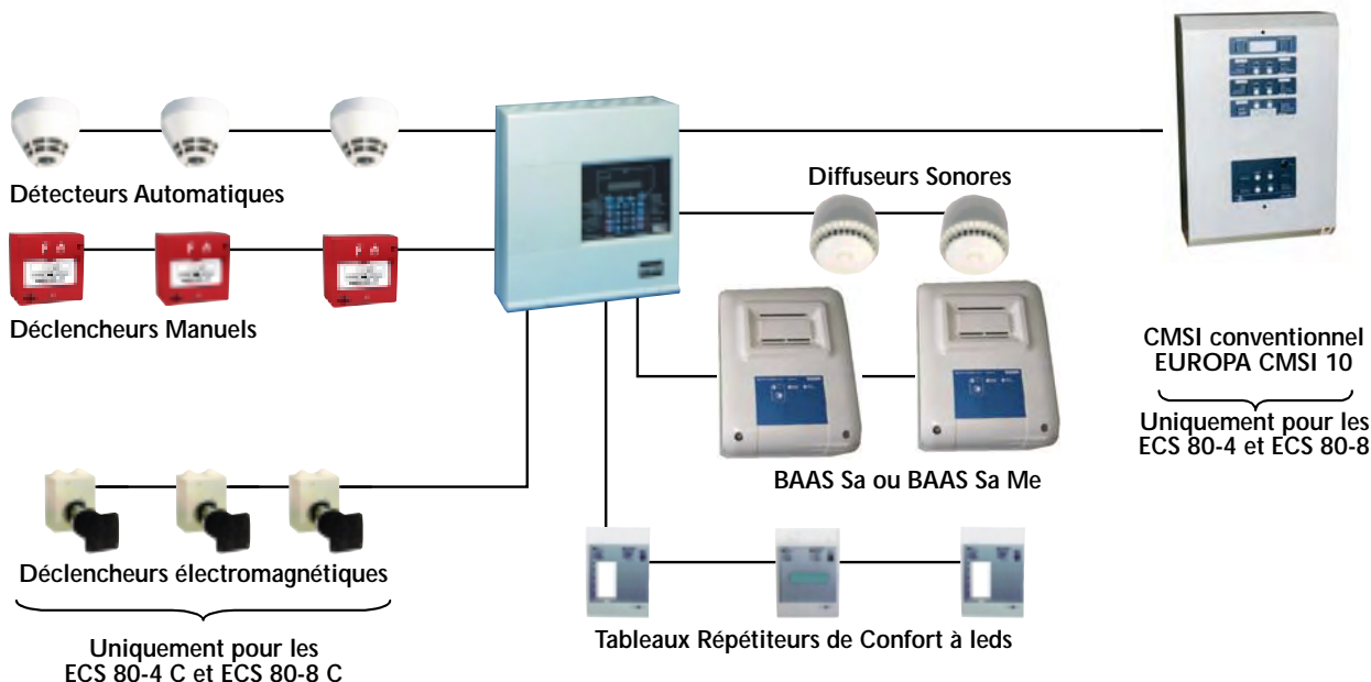
Architecture d'un système de détection incendie conventionnel
